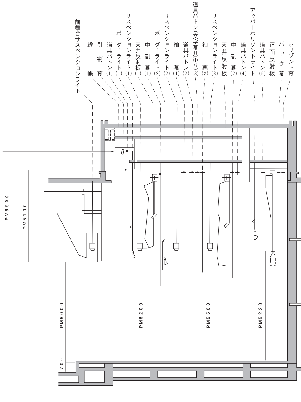
舞台断面図
